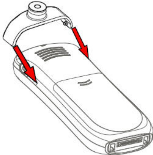
Рисунок 9: Привинтите шарнирный зажим в нужном месте
