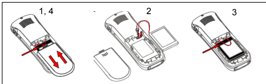
Рисунок 7: Сменная батарея
