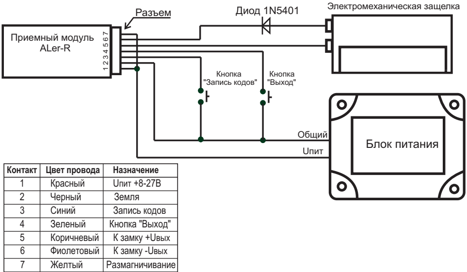
Рис.2 Схема подключения приемного устройства ALer-R к электромеханической защелке.
