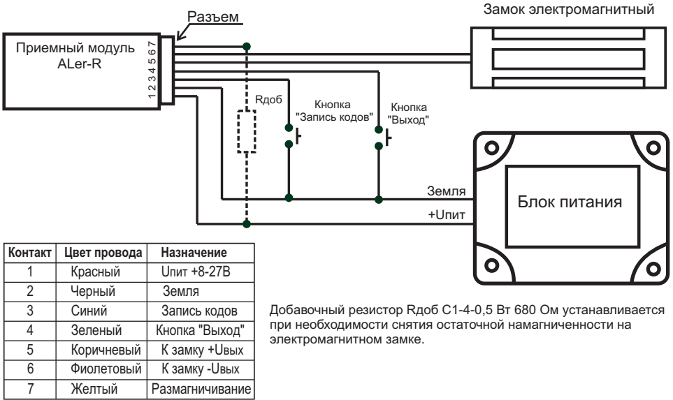
Рис1. Схема подключения приемного устройства ALer-R к электромагнитному замку.
