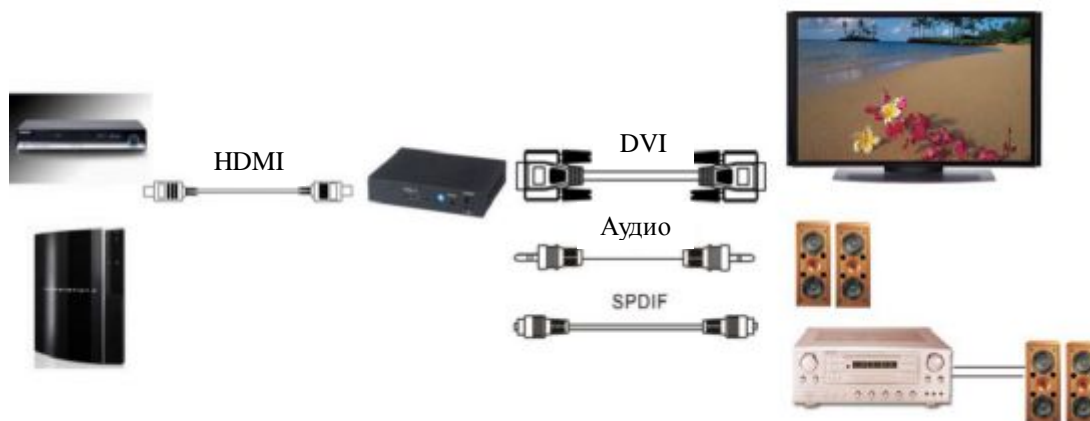
Рис.2 Схема подключения HD01
