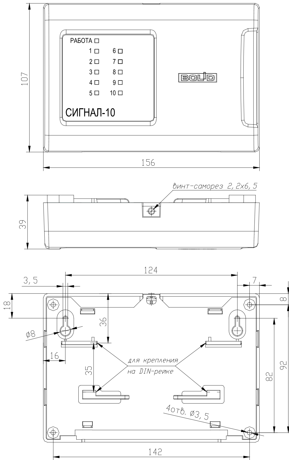
Рисунок 2. Габаритные и установочные размеры блока Сигнал-10
