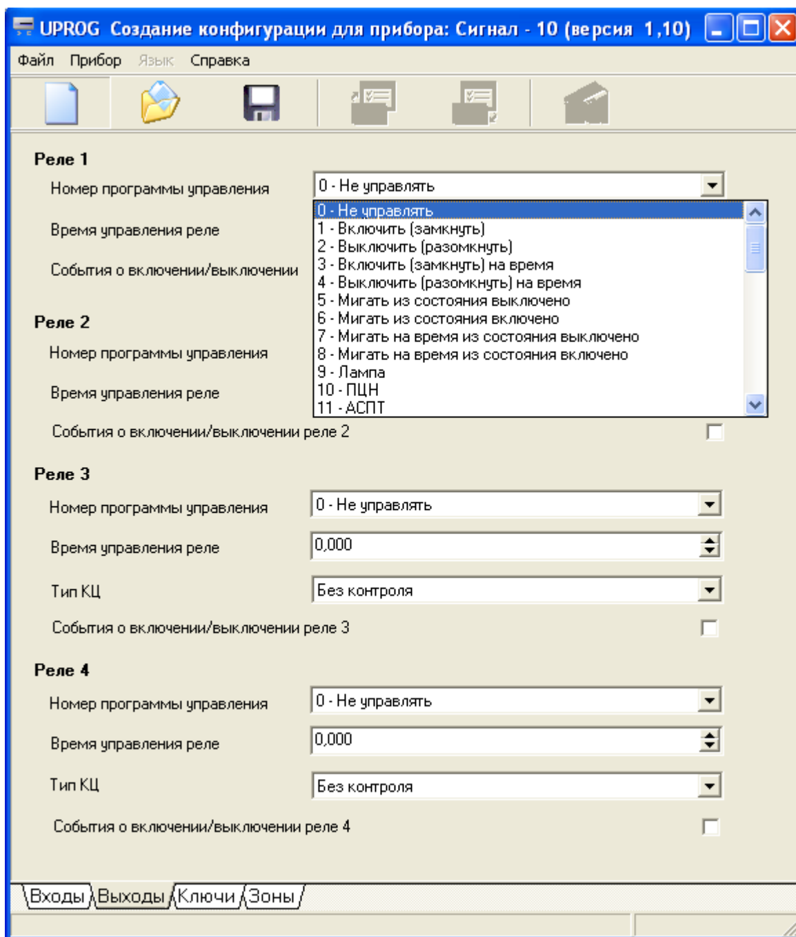
Рисунок 16. Программирование релейных выходов блока Сигнал-10
