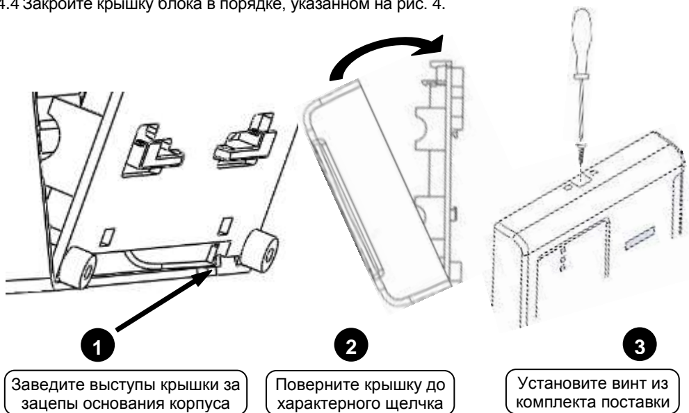
Рисунок 4. Установка крышки блока
