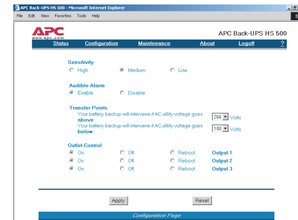
Рисунок 16. Окно настройки
