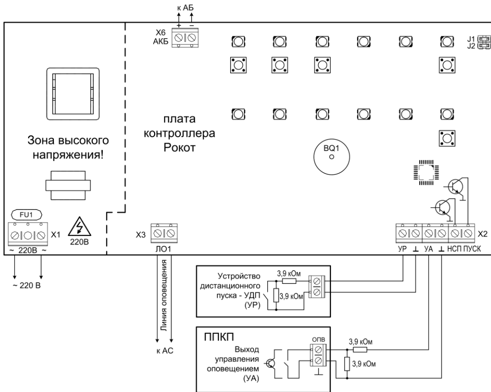
Рис.А1 Плата контроллера и схема внешних подключений прибора «Рокот»
