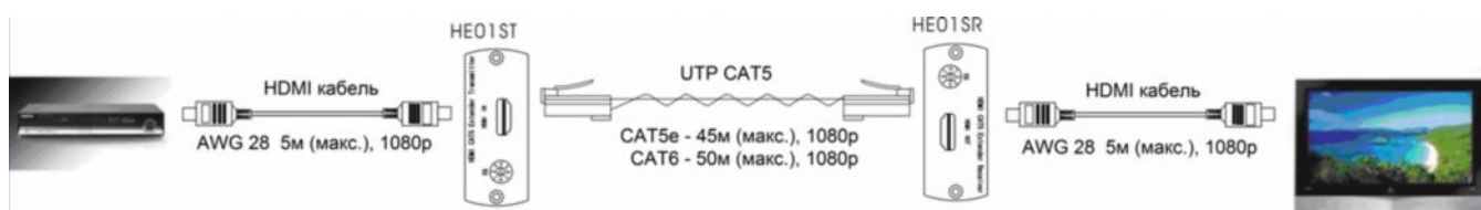
Рис.2 Структурная схема подключения
