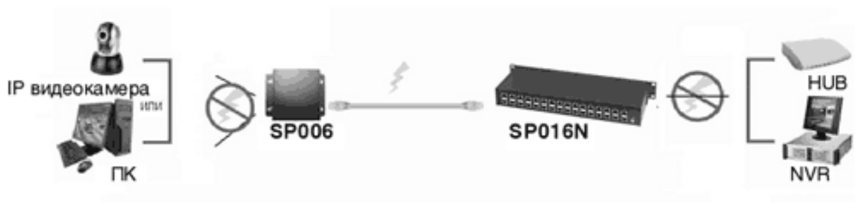
Рис.2 Подключение SP016N .
