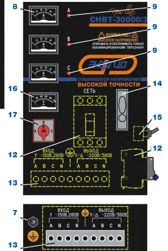
Рис. 7. Модели SNBT-9000/3...60000/3 Передняя панель – сверху. Задняя панель – внизу.
