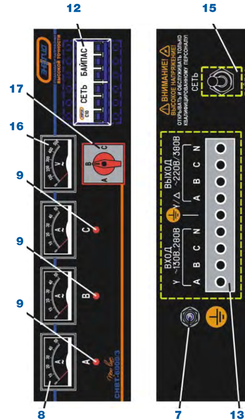
Рис. 6. Модели SNBT-4500/3, 6000/3 Передняя панель – слева. Задняя панель – справа
