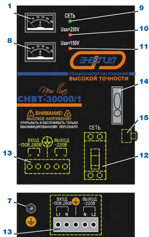
Рис. 5. Модели SNBT-15000/1...30000/1 Передняя панель – сверху. Задняя панель – внизу.
