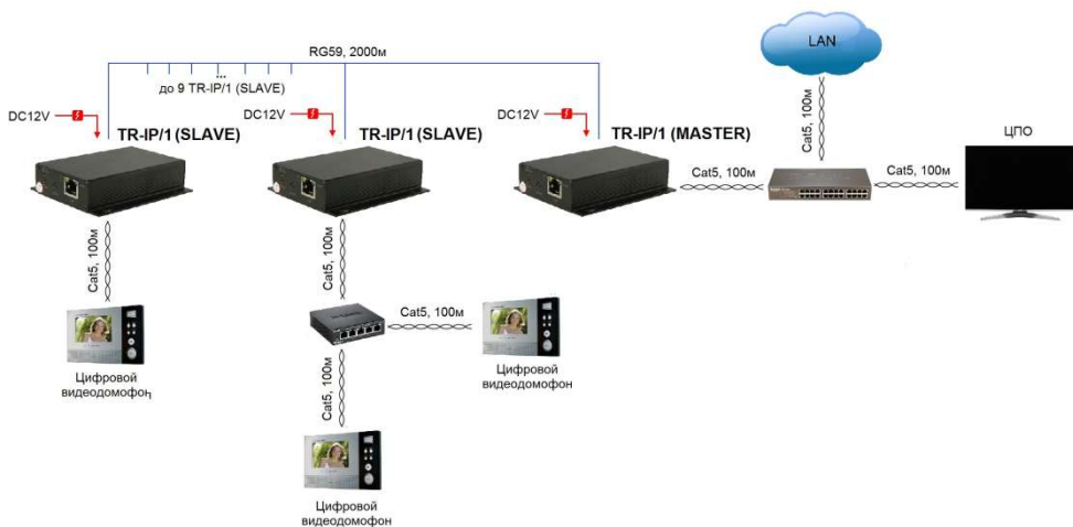
Рис. 6 Схема подключения TR-IP/1(MASTER) и TR-IP/1(SLAVE) для организации ЦПО.
