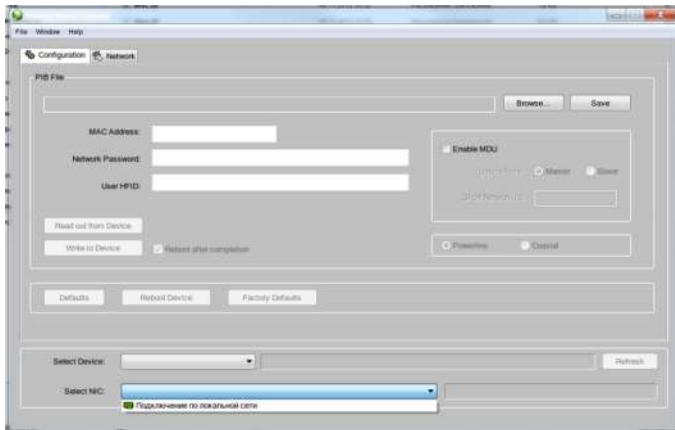
Рис. 9 Вкладка Network
