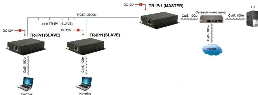
Рис. 3 Схема подключения TR-IP/1(MASTER) и TR-IP/1(SLAVE) для организации удаленного сегмента сети.
