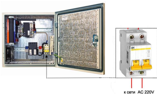
Рис.4 Точка подключения уличной станции к сети 220V переменного тока на примере модели OS-44VB1
