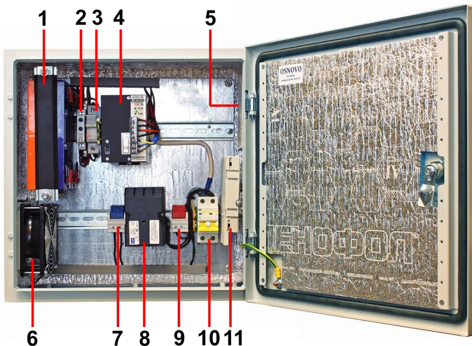
Рис.2 Уличная станция с системой обогрева, проточной вентиляции и резервным питанием, внутренние компоненты, на примере модели OS-44VB1
