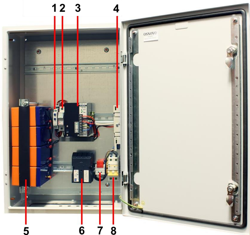
Рис.2 Уличная станция с системой обогрева и резервным питанием, внутренние компоненты, на примере модели OS-46TB1
