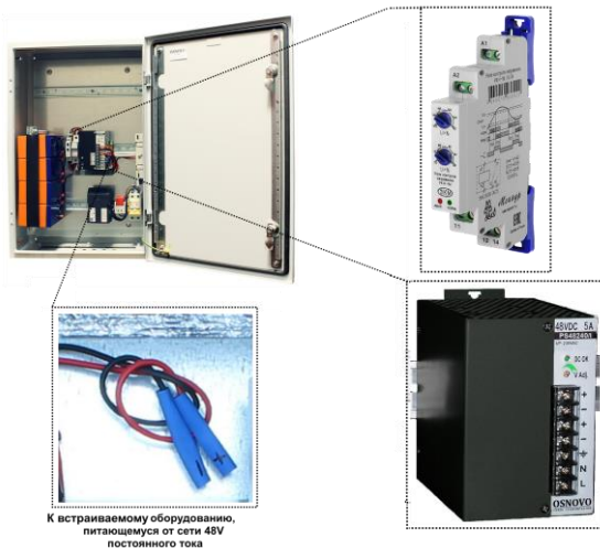
Рис.4 Точка подключения оборудования к 48V для моделей уличных станций с установленным БП и резервным питанием на примере модели OS-46TB1
