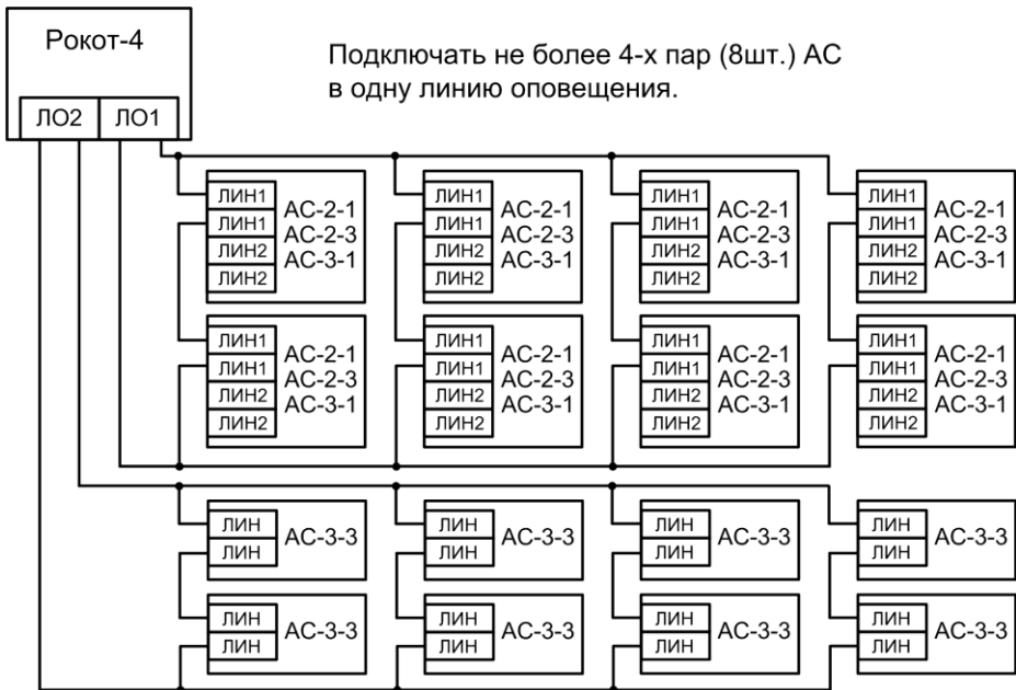
Рис.А2 Схема подключения акустических систем «АС-2-1», «АС-2-3», «АС-3-1» и «АС-3-3» (параллельно-последовательное соединение АС)
