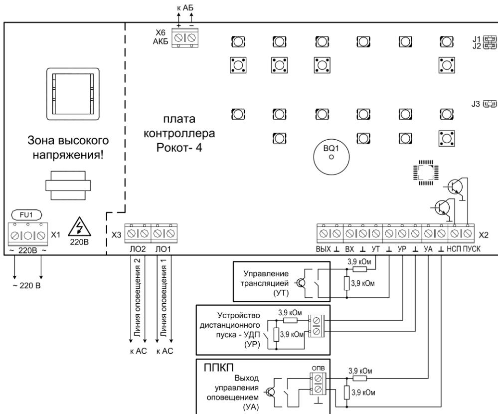
Рис.А1 Плата контроллера и схема внешних подключений прибора «Рокот-4»
