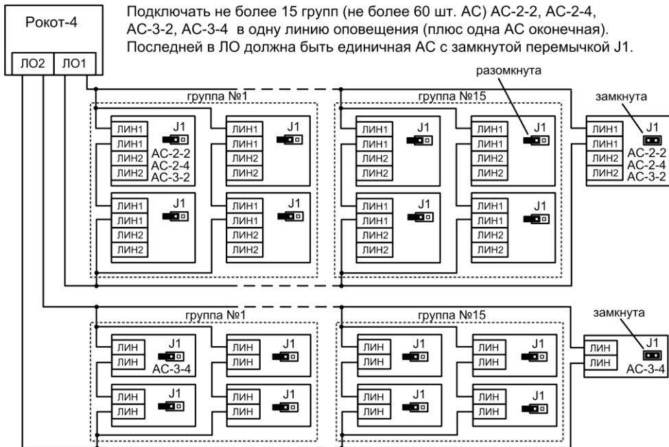
Рис.А4 Схема подключения акустических систем «АС-2-2», «АС-2-4», «АС-3-2» и «АС-3-4» (параллельное соединение групп АС)
