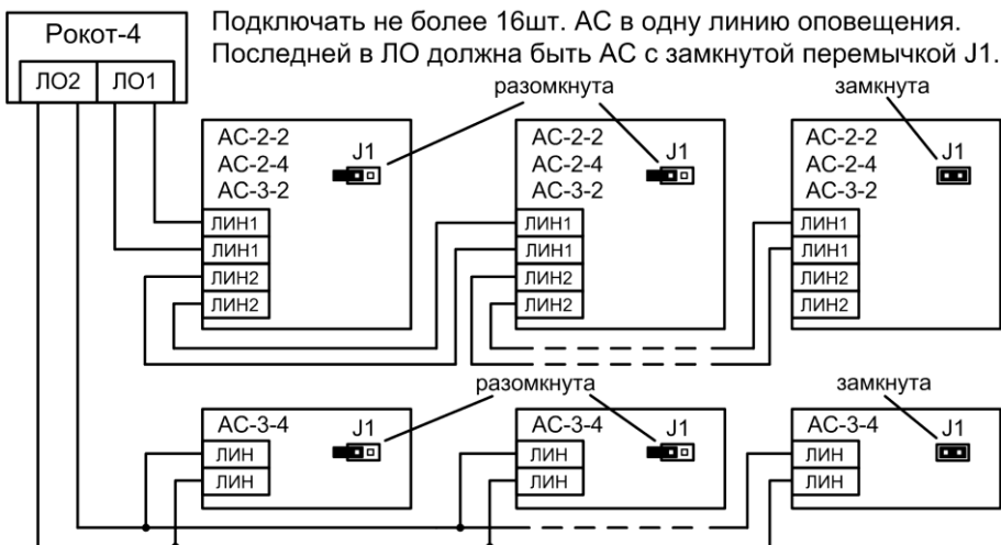
Рис.А3 Схема подключения акустических систем «АС-2-2», «АС-2-4», «АС-3-2» и «АС-3-4» (параллельное соединение АС)
