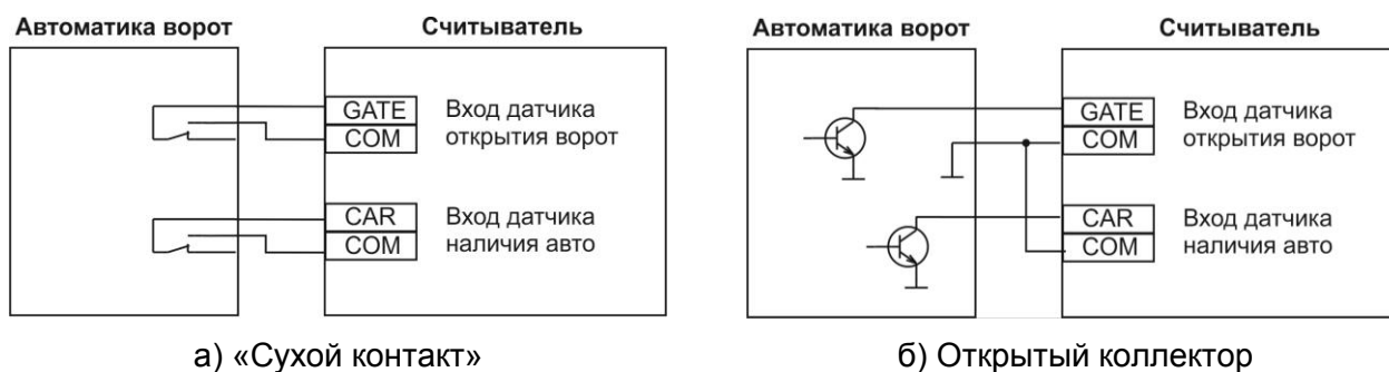
Рисунок 19. Подключение датчиков автоматике (один канал)
