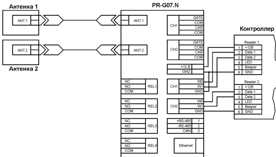
Рисунок 13. Интерфейс Wiegand
