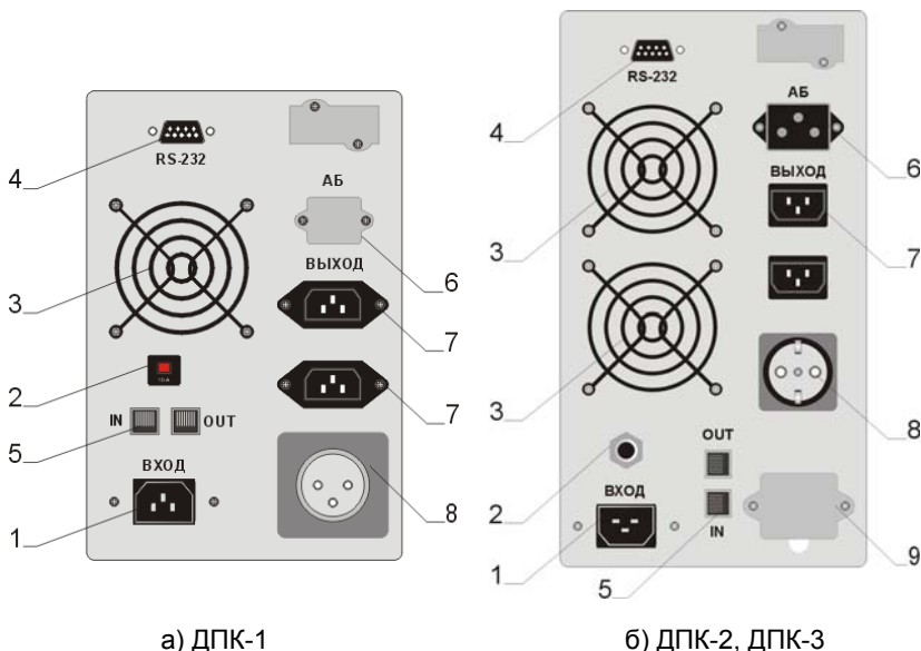
Рис. 2 Задняя панель блока ИБП:
