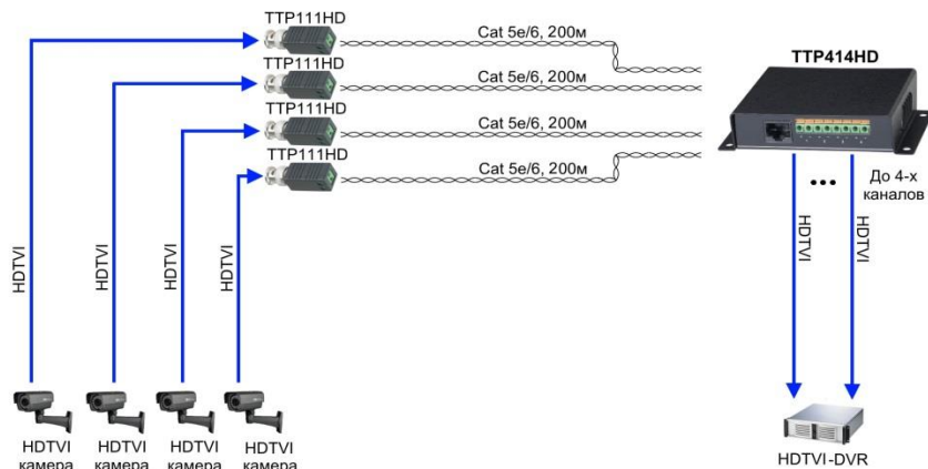
Рис. 4 Схема подключения приемопередатчика TTP414HD и приемопередатчиков TTP111HD для работы с HDTVI-видеокамерами
