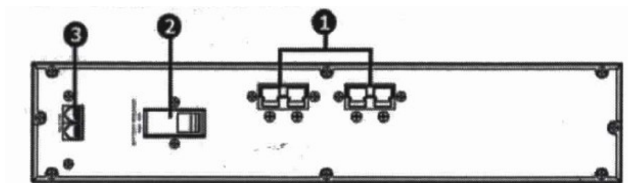
Рис.1 Задняя панель батарейного блока BFR96-9E
