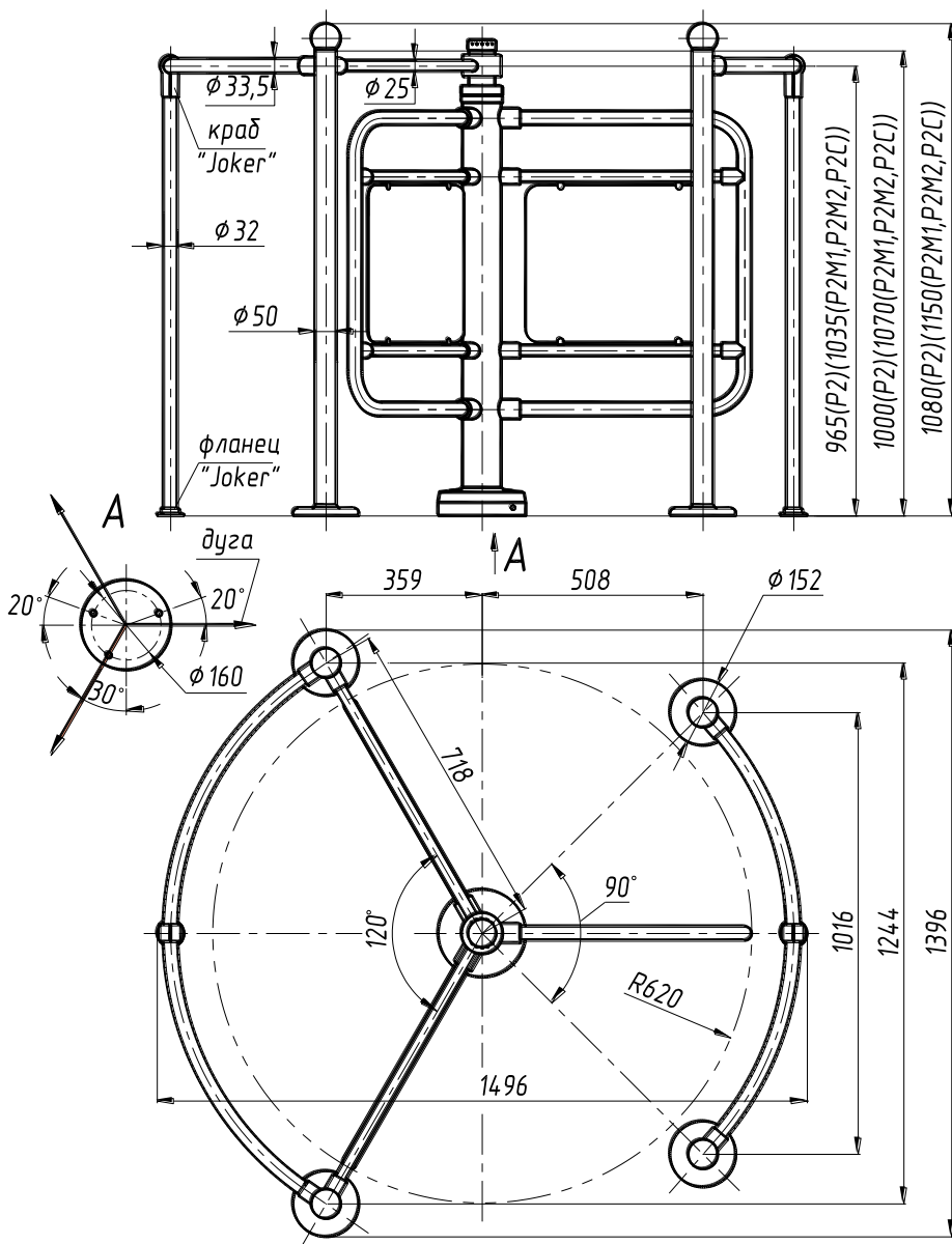
Установочные размеры роторных турникетов трехлопастных и ограждения «Люк В) I-P)
