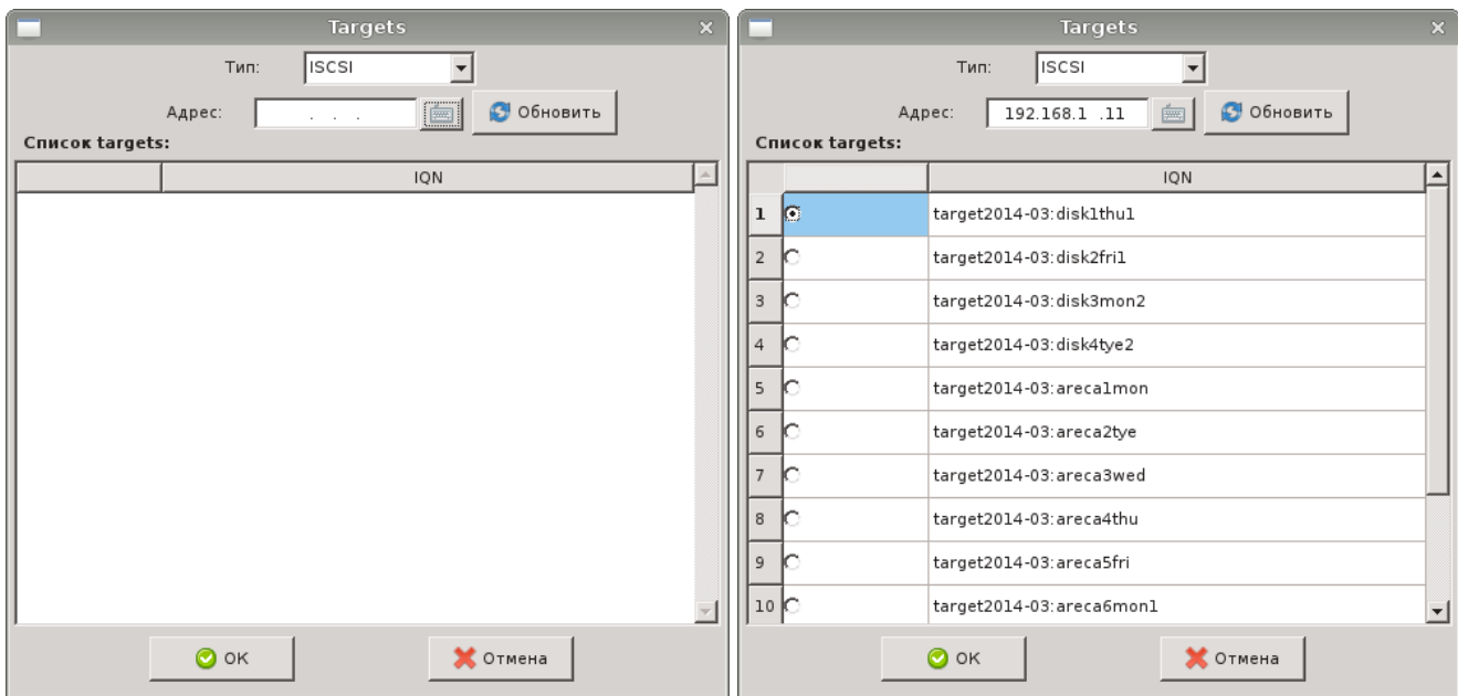
а) б) Рисунок 34 - Окно настройки подключения сетевого хранилища: а – пустое, б – с выбранным target
