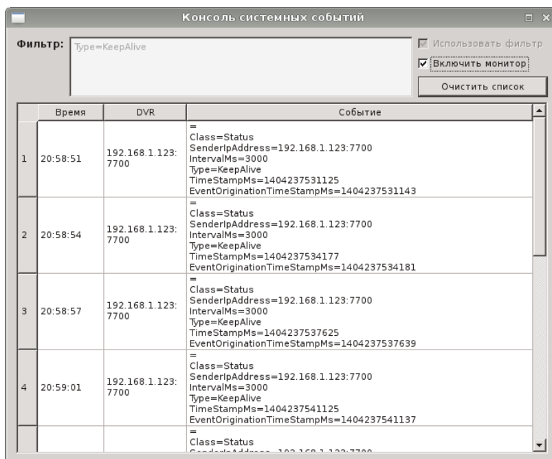
Рисунок 80 - Консоль системных событий с включенным фильтром и монитором
