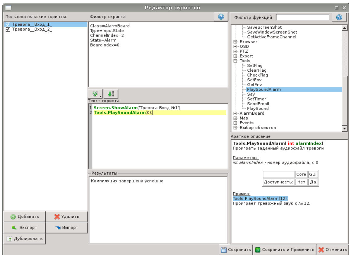
Рисунок 81 - Окно «Редактор скриптов»
