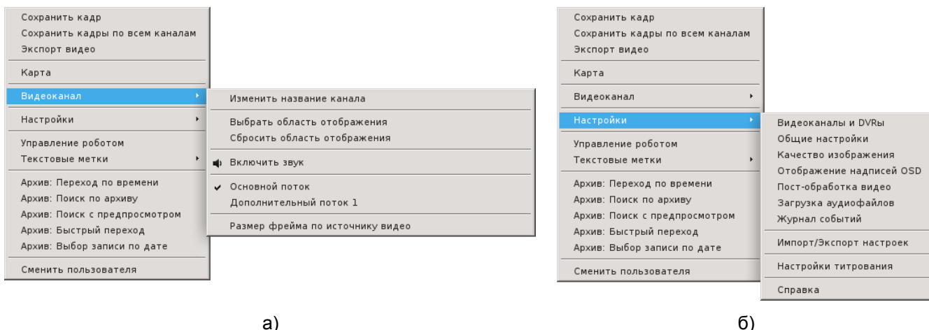
Рисунок 2 – Основное контекстное меню в режиме «Live»: а - подменю «Видеоканал», б - подменю «Настройки».
