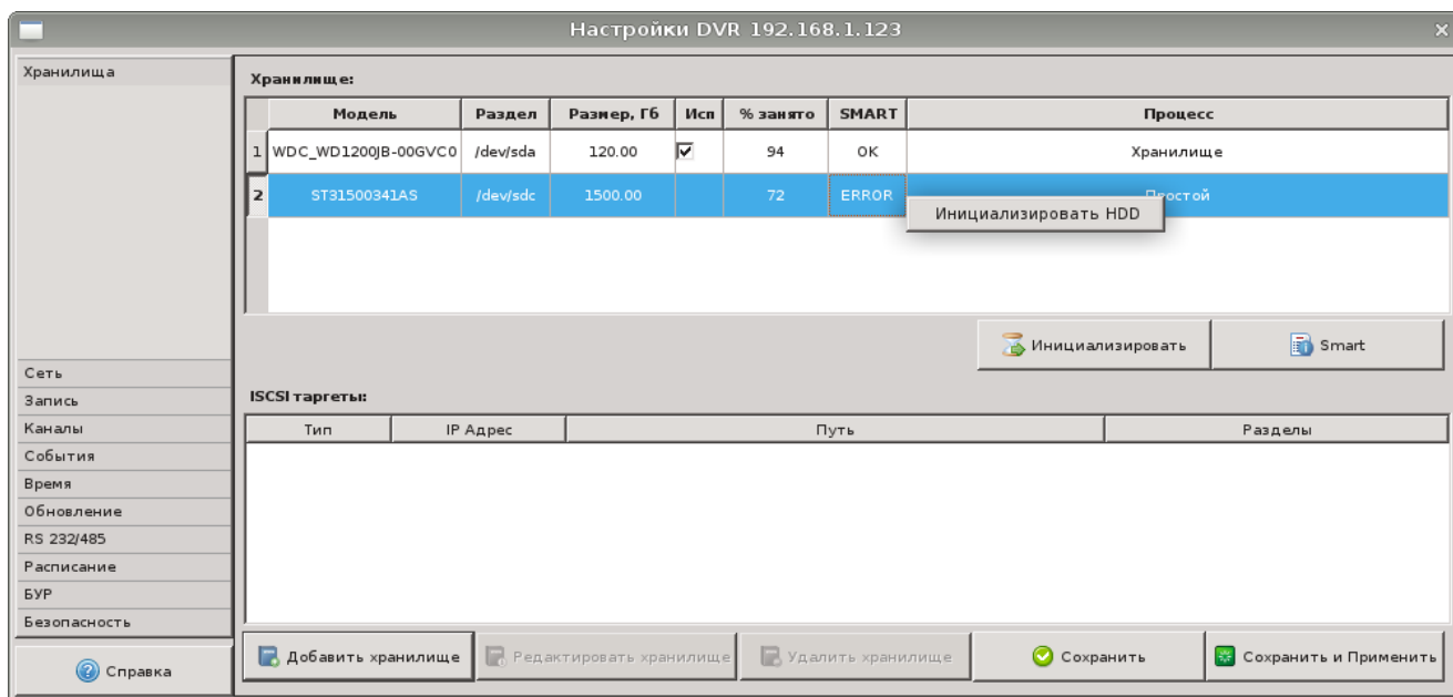
Рисунок 28 - Контекстное меню окна настройки DVR, вкладка «Хранилища»
