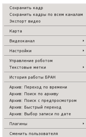
Рисунок 118 - Вид контекстного меню при авторизации пользователя Guest
