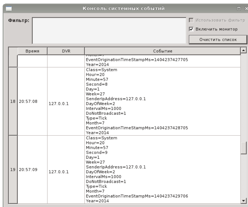
Рисунок 79 - Консоль системных событий с включенным монитором
