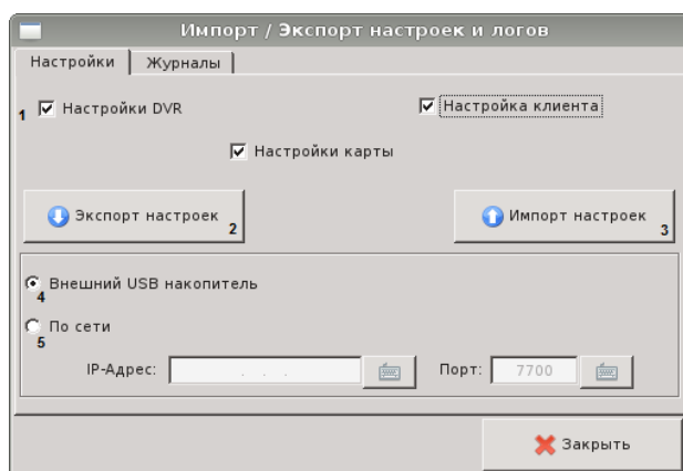
Рисунок 188 - Окно импорта/экспорта настроек и логов, вкладка «Настройки»
