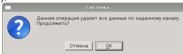
Рисунок 56 - Предупреждающее сообщение
