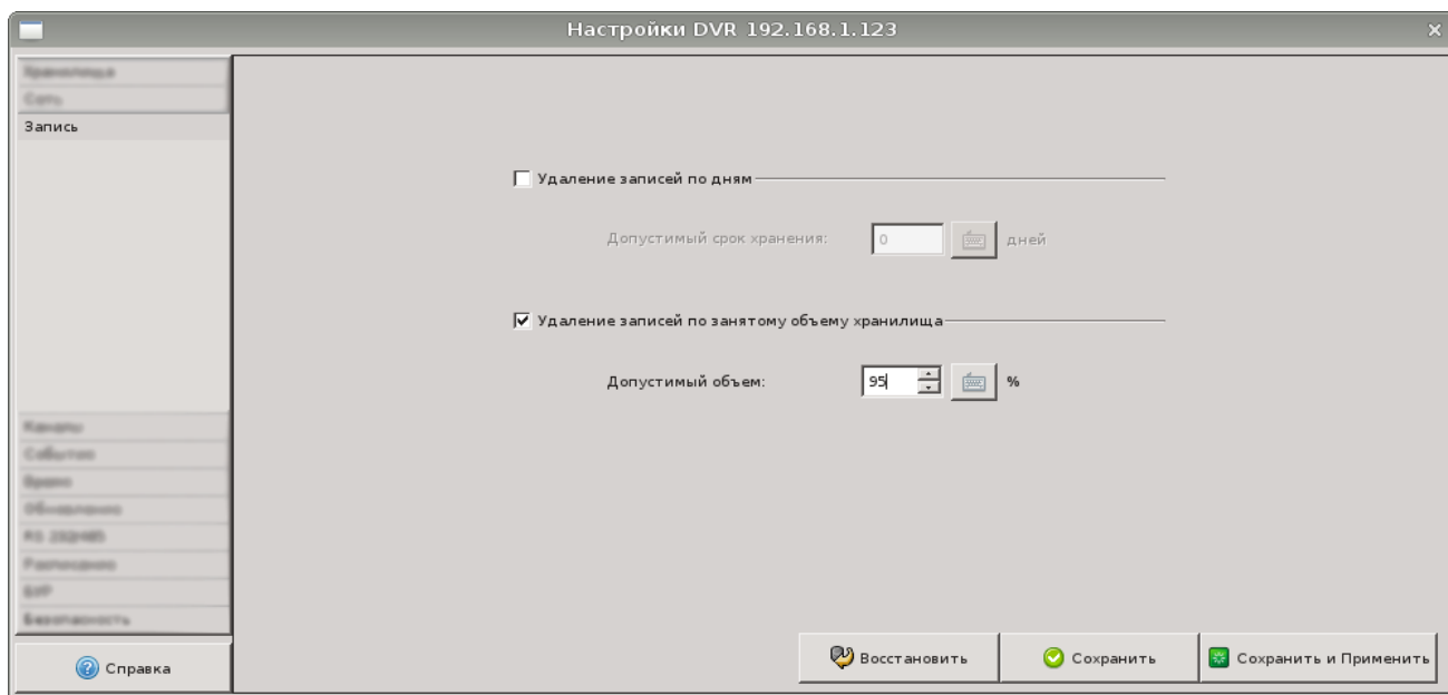
Рисунок 39 - Окно настройки DVR, вкладка «Запись»
