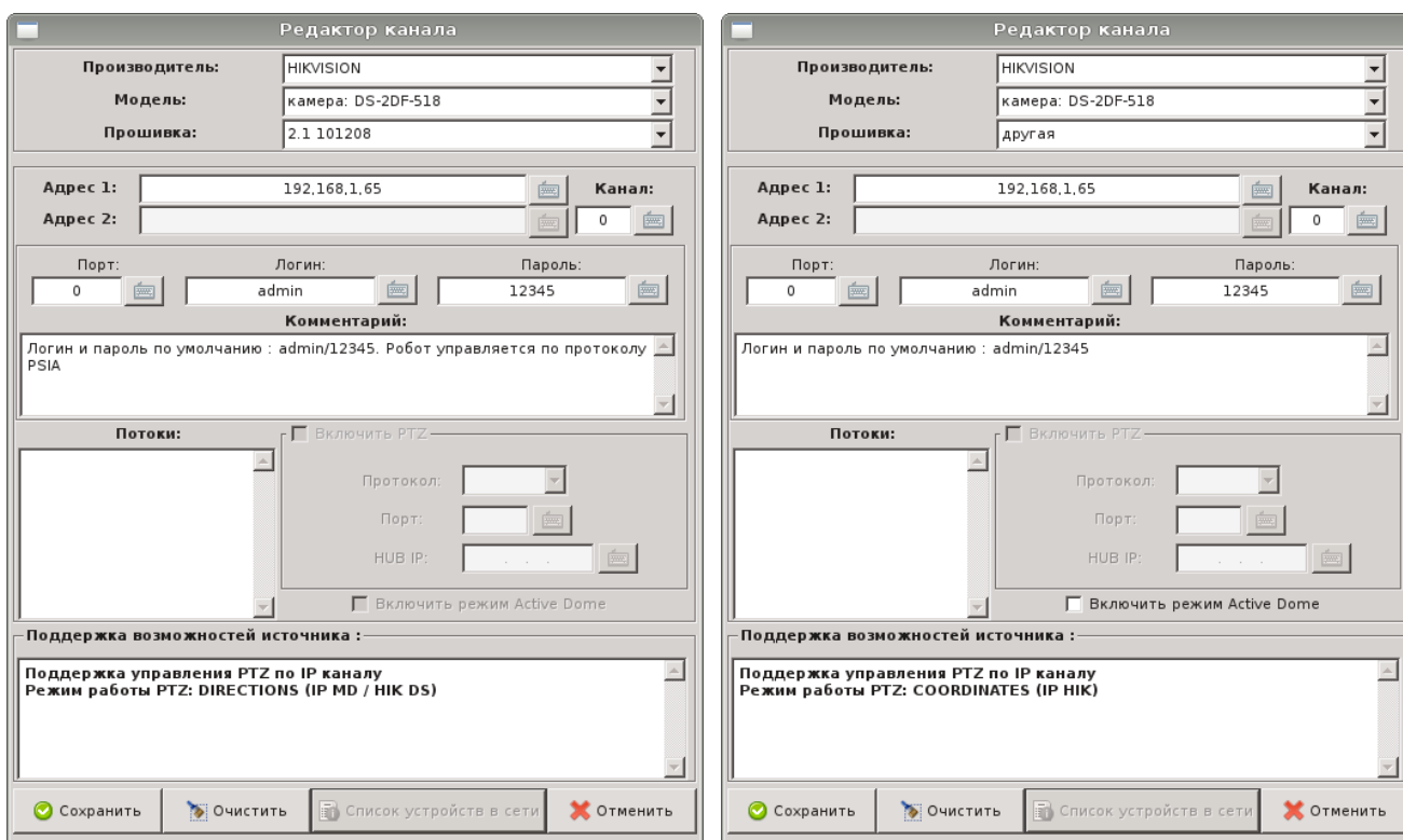
Рисунок 177 - Окно редактора канала, настройка параметров PTZ: а) режим «DIRECTIONS (IP MD / NIK DS)», б) режим «COORDINATES (IP NIK)»
