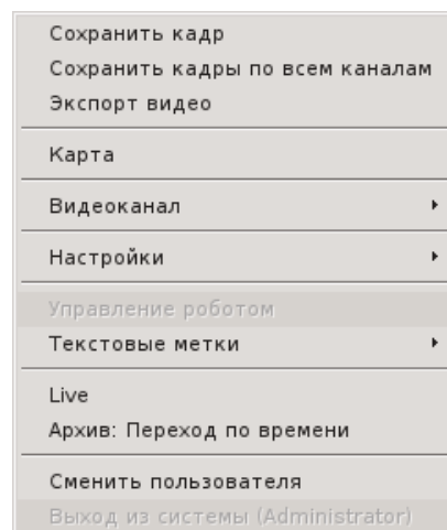
Рисунок 7 - Основное контекстное меню под учетной записью «Administrator»:
