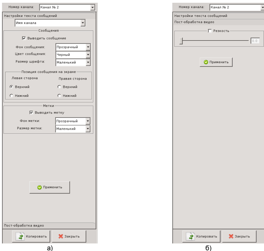
Рисунок 96 - Боковая панель настройки: а – текста сообщений, б - пост-обработки видео
