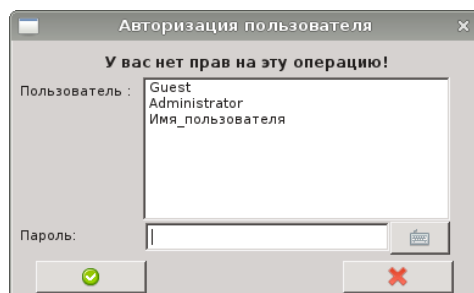
Рисунок 114 - Окно авторизации
