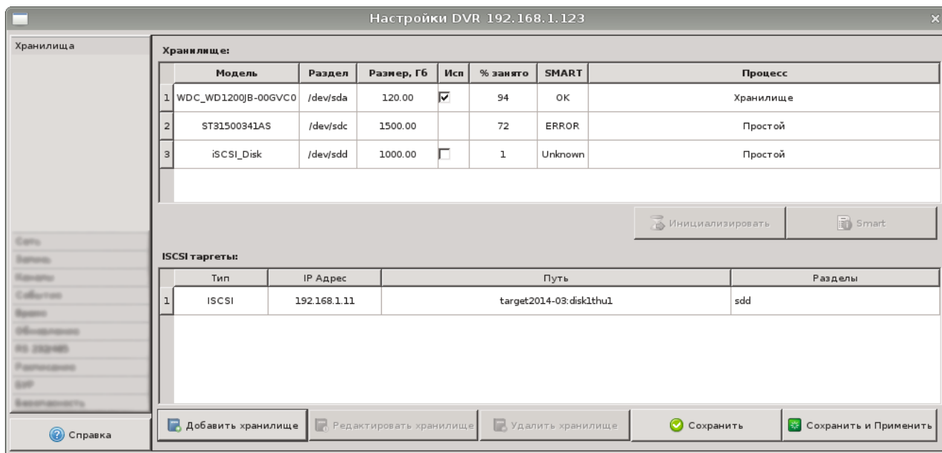
Рисунок 36 - Окно настройки DVR, вкладка «Хранилища» добавлено сетевое хранилище
