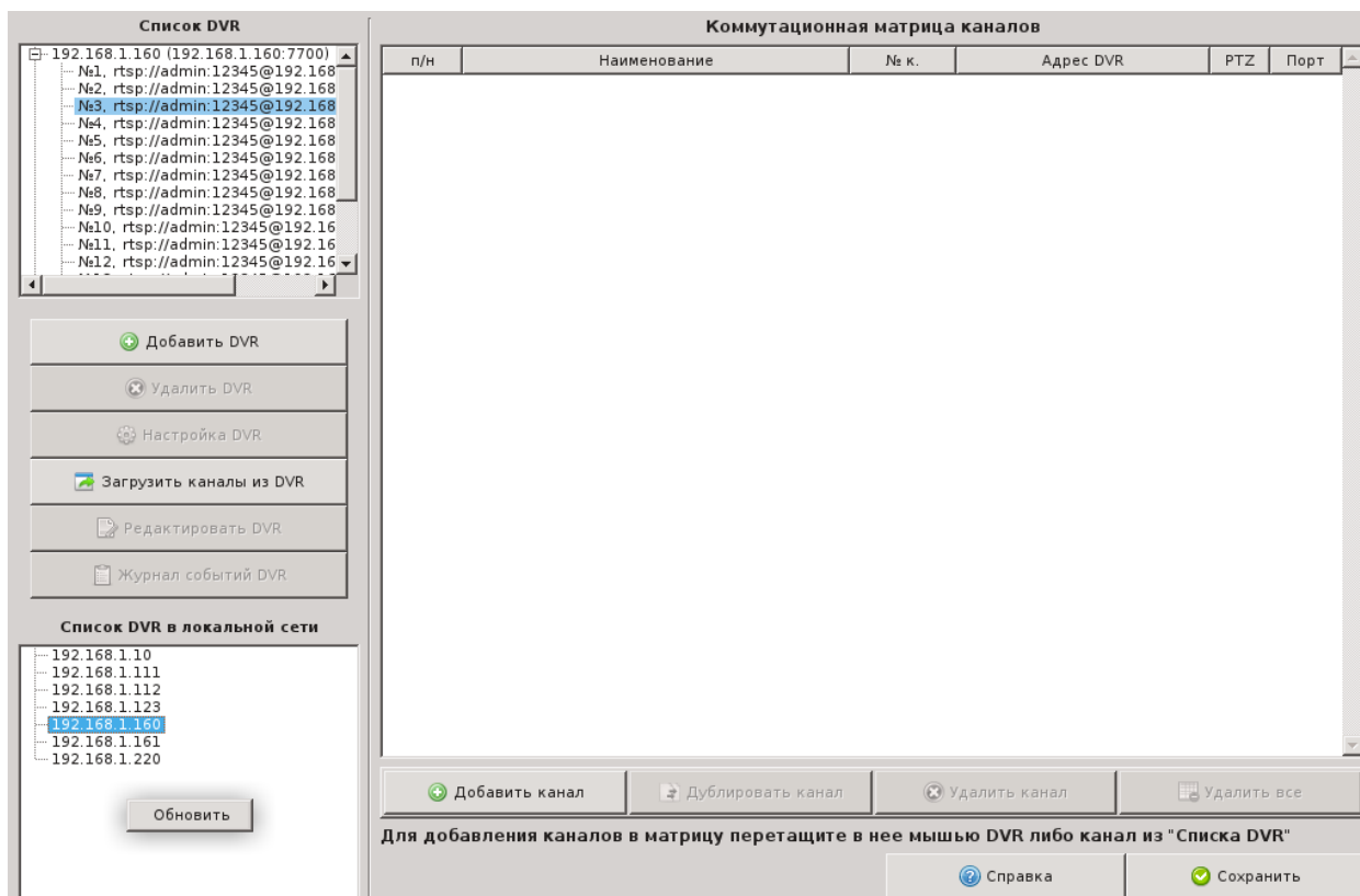
Рисунок 16 - Окно «Настройка видеоканалов и DVR-ов», пункт контекстного меню «Обновить»
